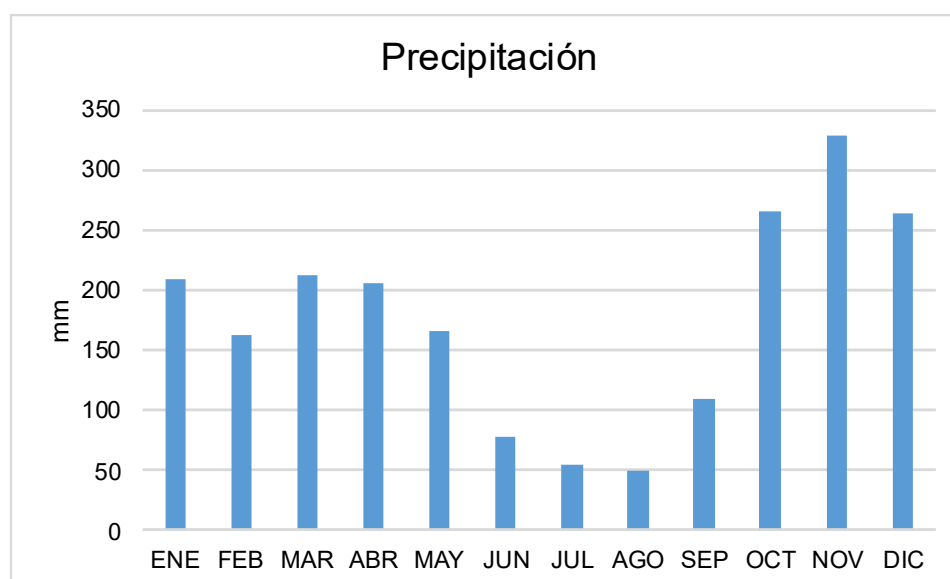
Figura 3 Precipitación media total departamento del Cauca
