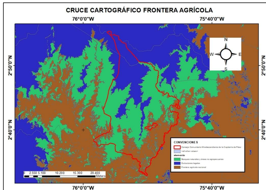
Mapa 10. Cruce cartográfico con la frontera agrícola
